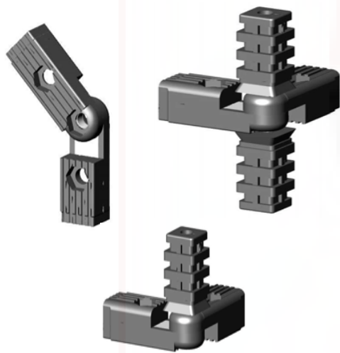
Gelenkverbinder ohne Kopf für unsichtbare Verbindungen
